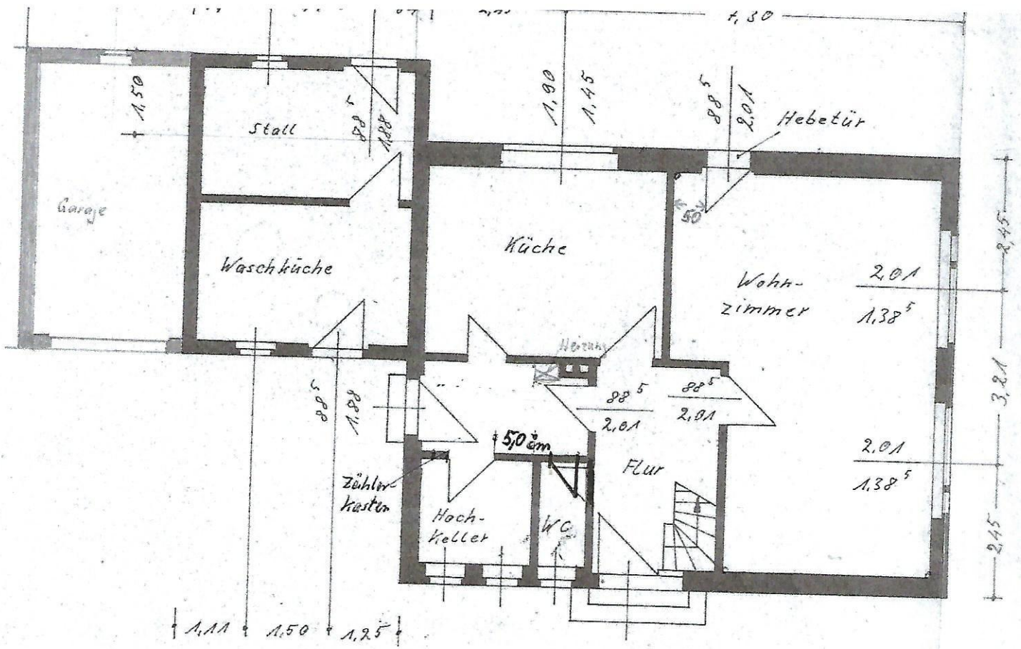
Erdgeschoss B
