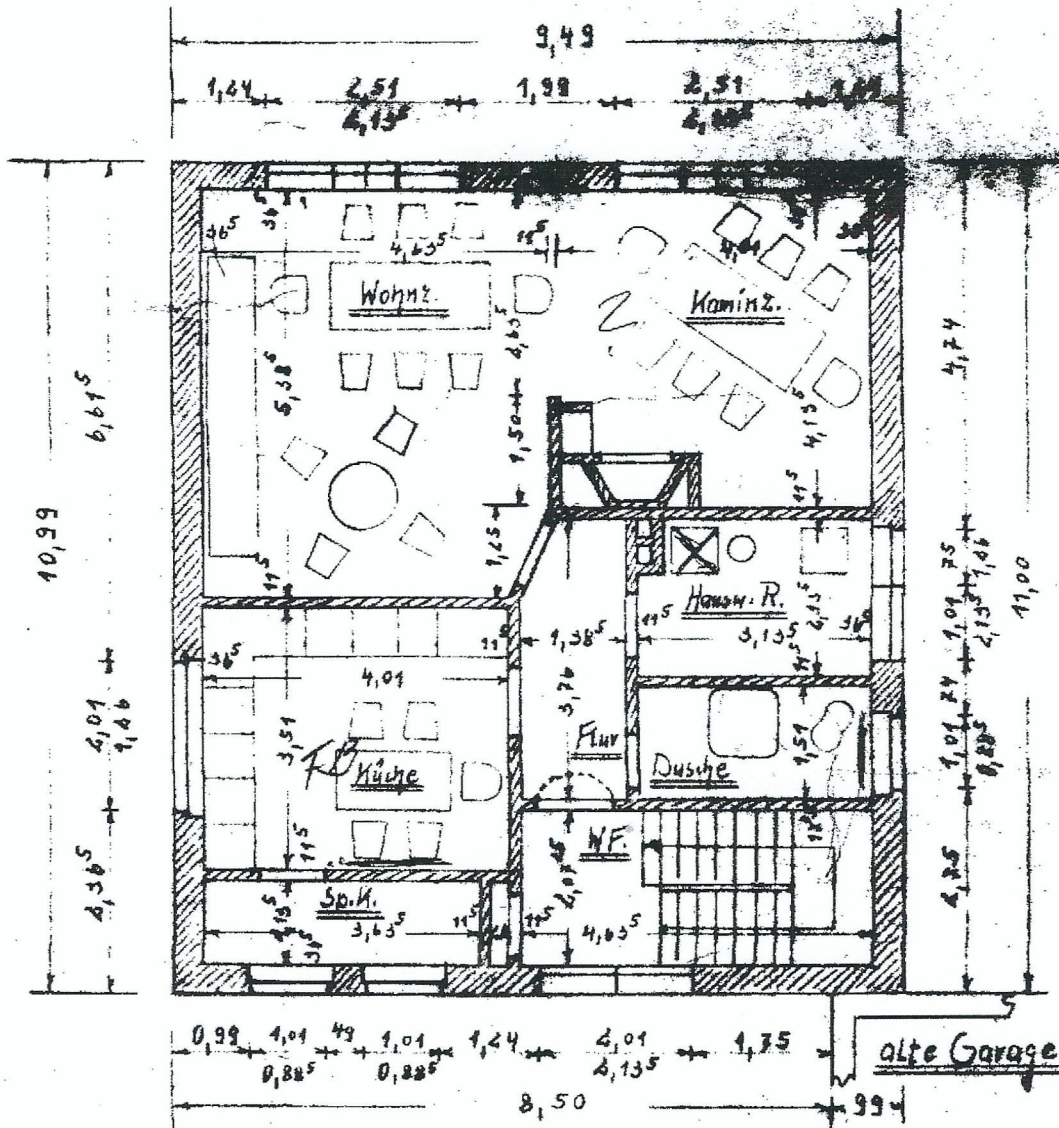
Grundriss M 1:100
