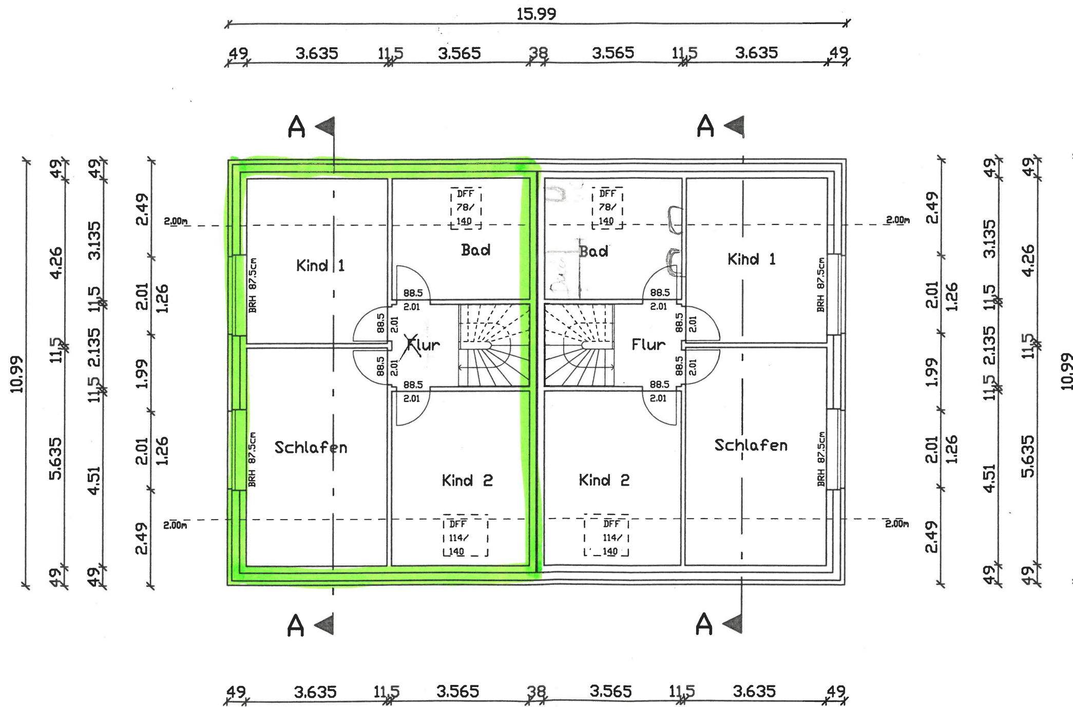
Dachgeschoss
