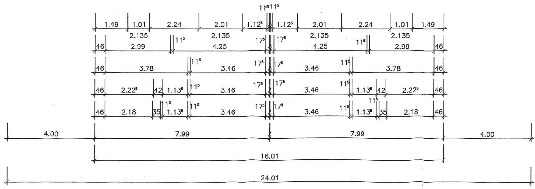
Grundriss
