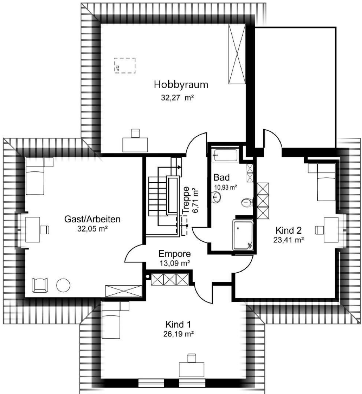
Dachgeschoss
