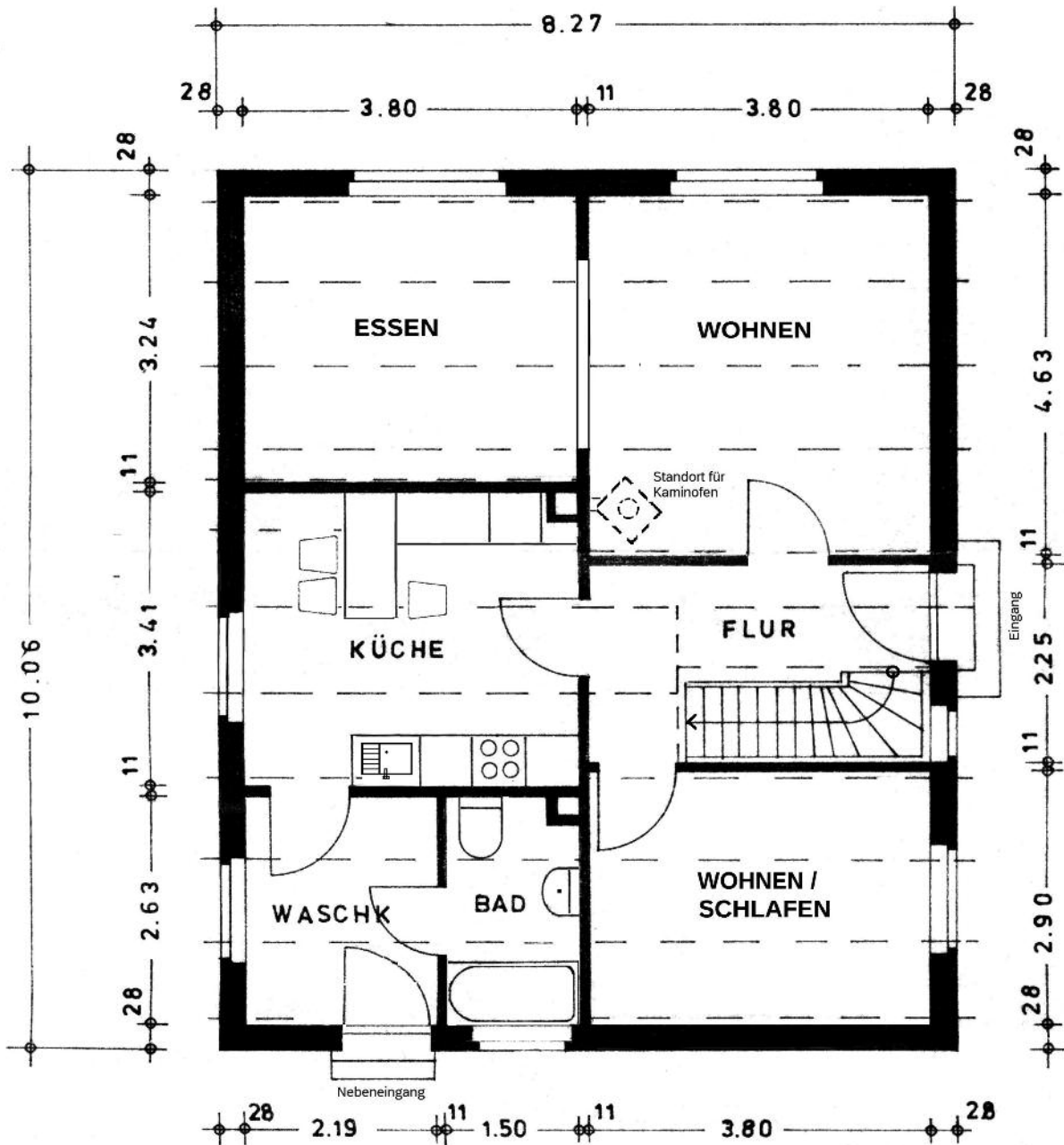
ERDGESCHOSS
