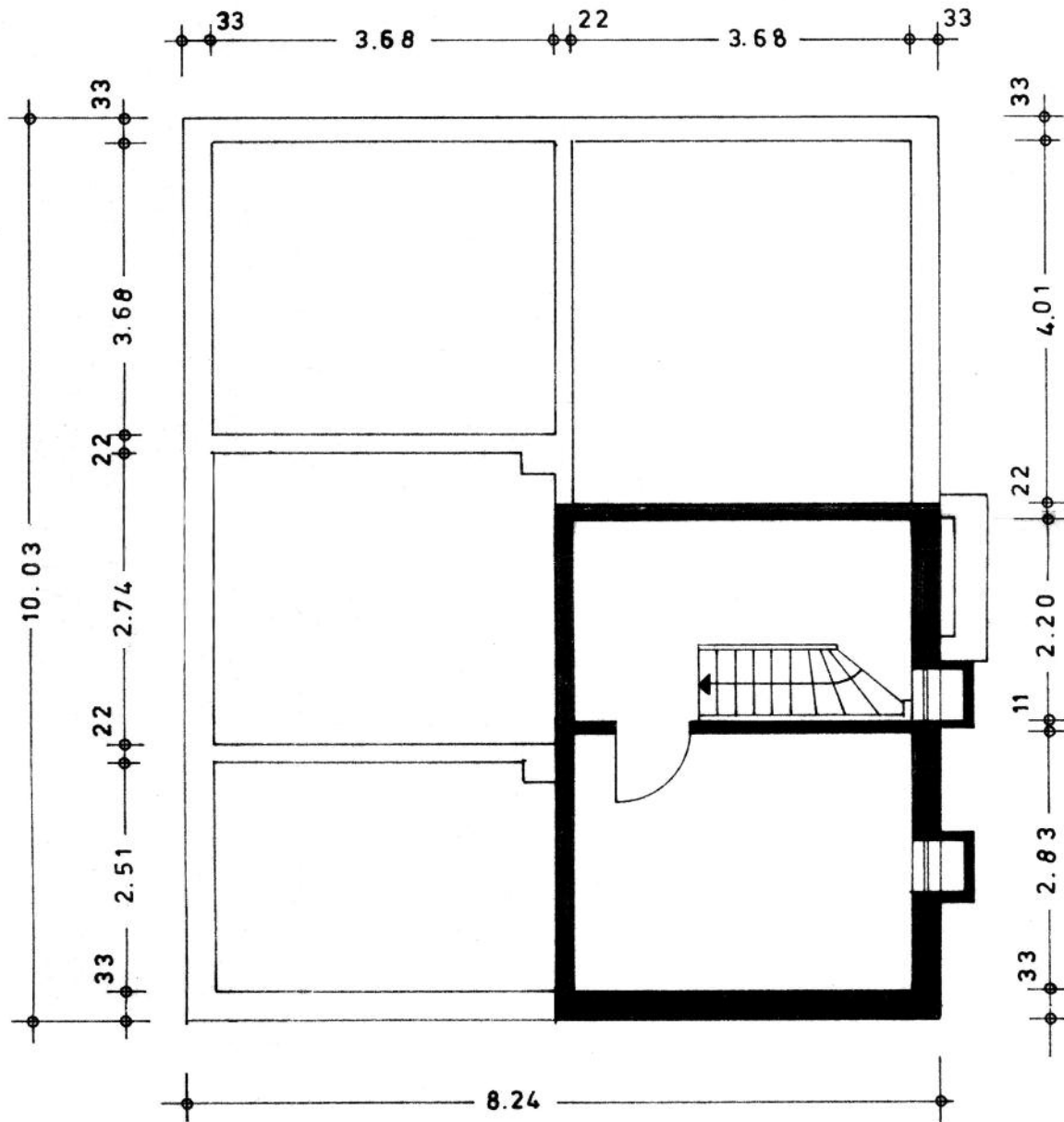
KELLER GESCHOSS
