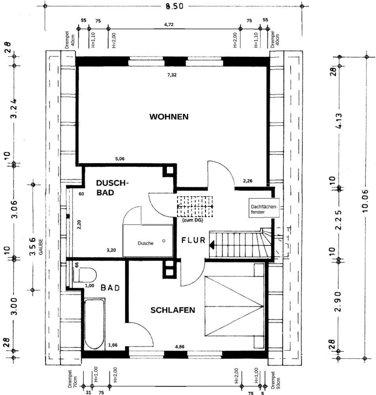
DACHGESCHOSS
