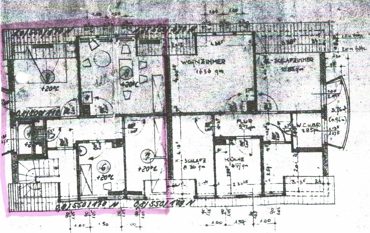
DACHGESCHOSS
