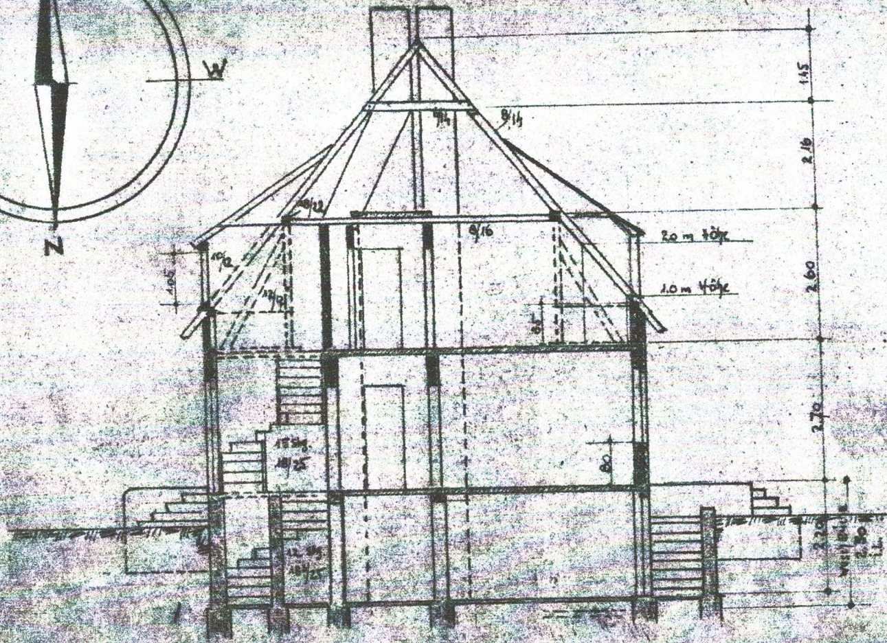
SCHNITT A-B
