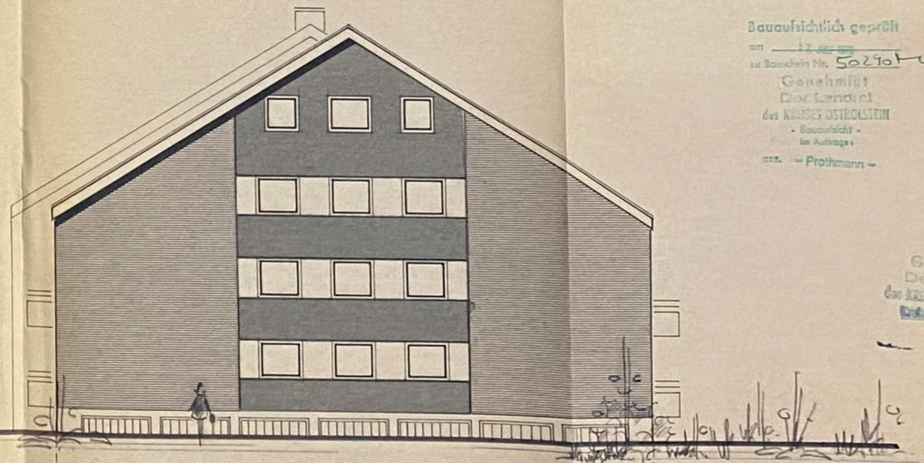
SÜD - ANSICHT
