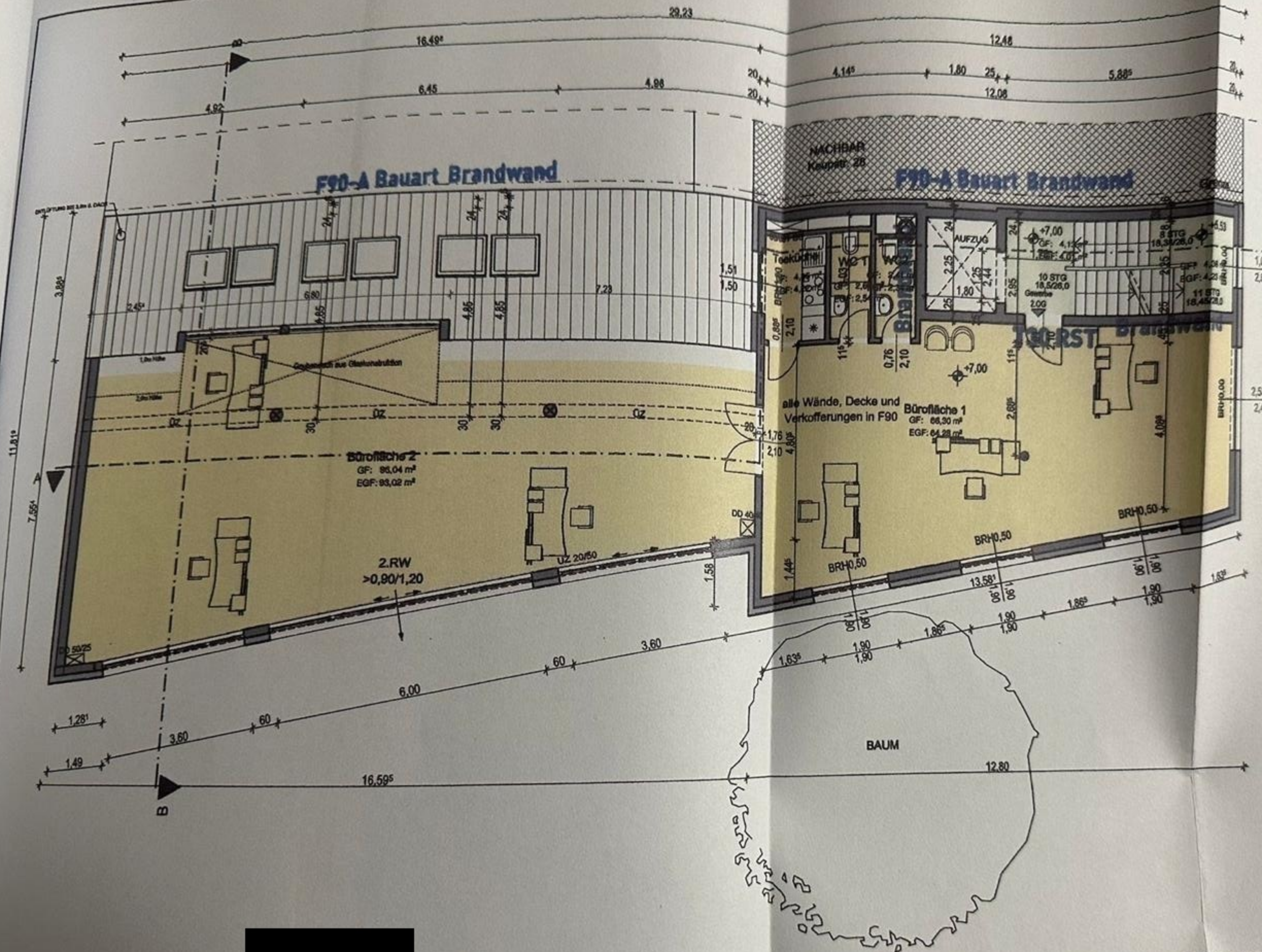
2. OBERGESCHOSS M: 1/100
