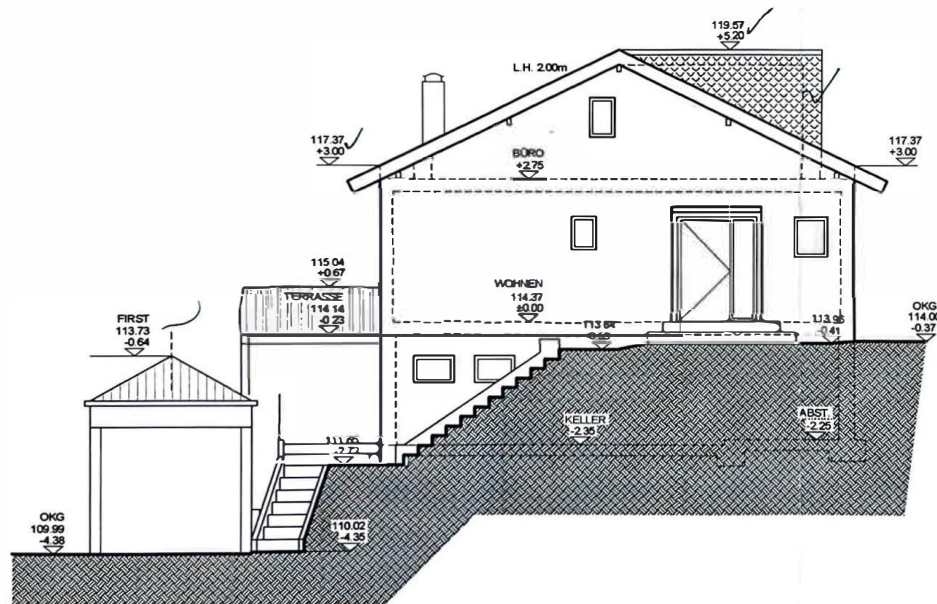
ANSICHT OST M 1:100
