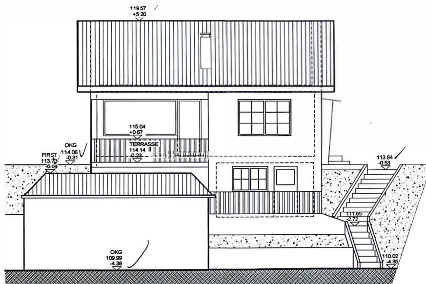
ANSICHT SÜD M 1:100
