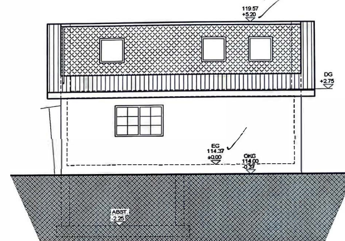
ANSICHT NORD M 1:100
