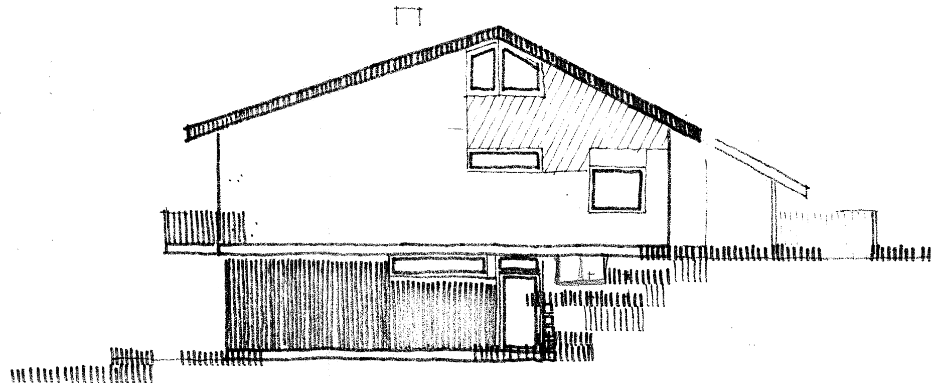
OSTEN 1:100
