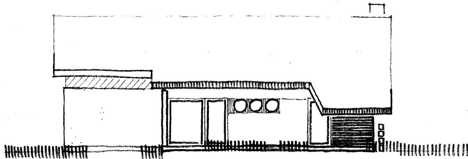
NORDEN 1:100
