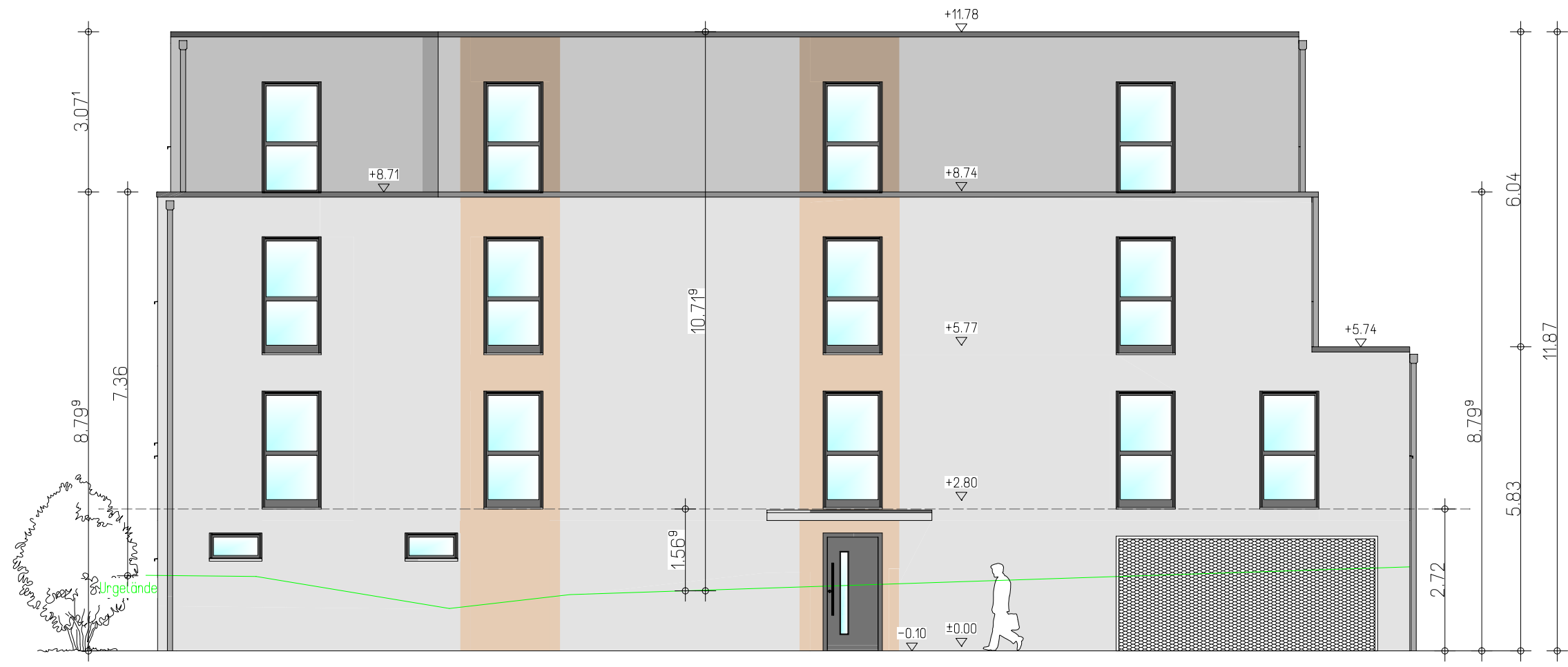
Ansicht Südwest
