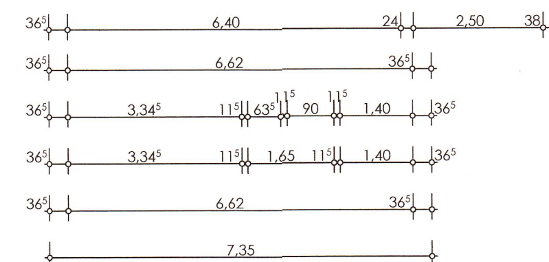
3. OBERGESCHOSS
