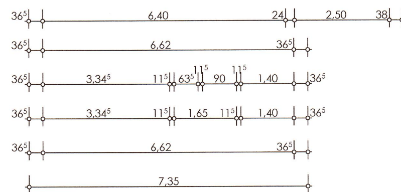
2. OBERGESCHOSS
