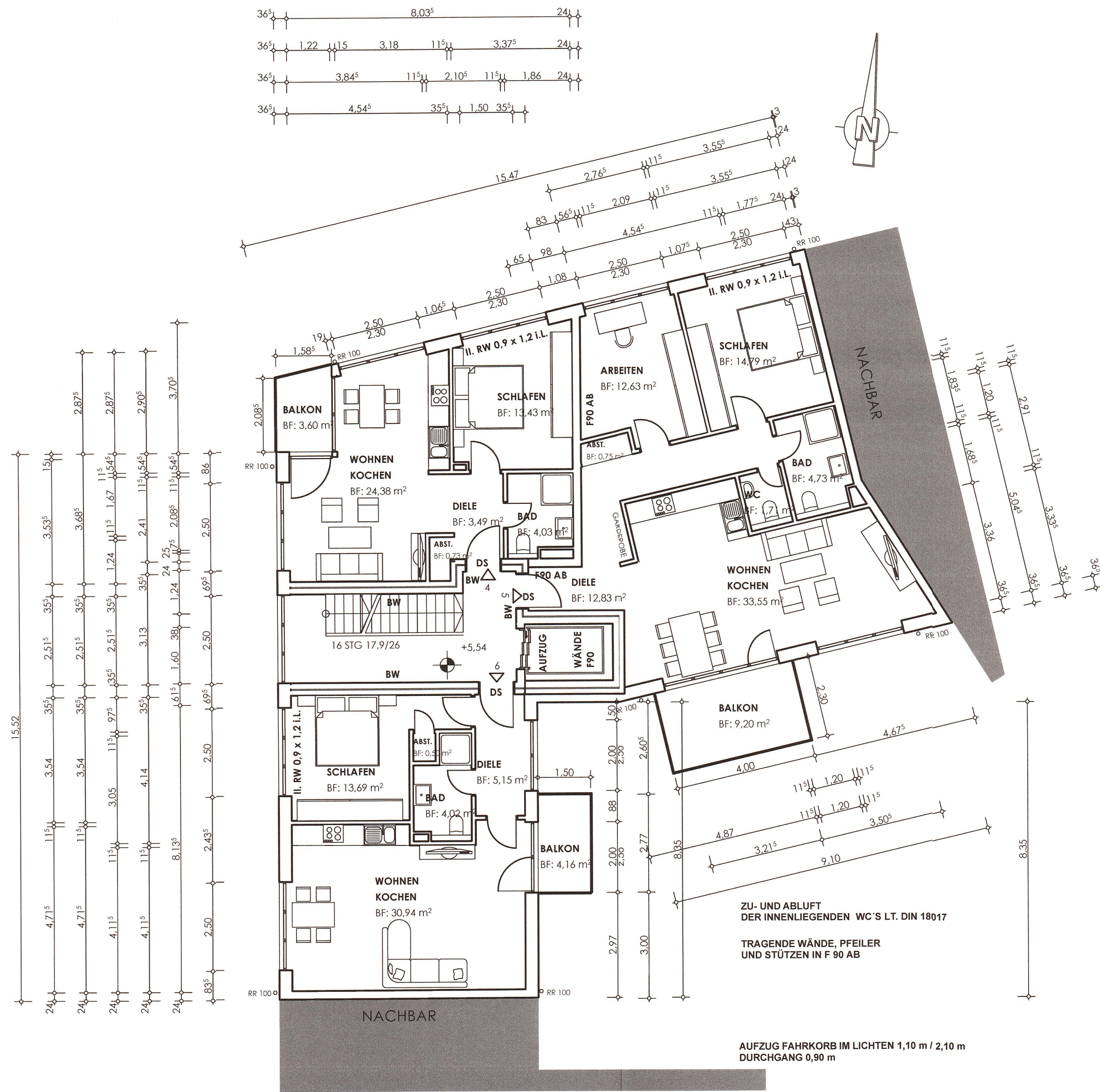
2. OBERGESCHOSS
