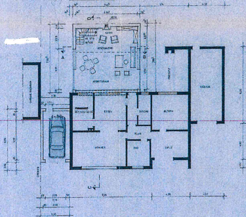
ERDGESCHOSS
