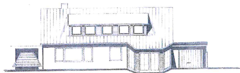
SÜD-OST-ANSICHT
