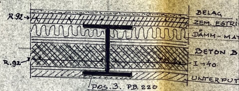
DETAIL POS. 1-2-3.
