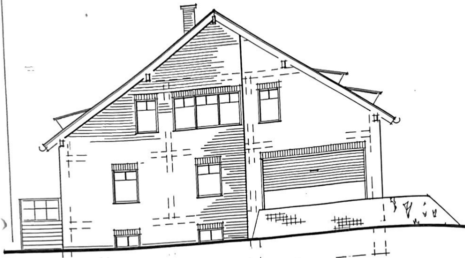
WESTANSICHT
