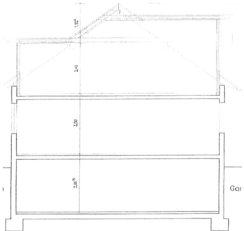
Schnitt
