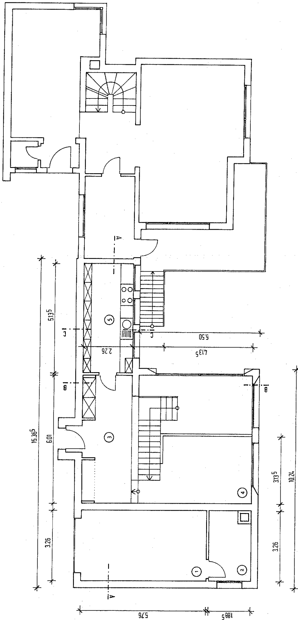
Grundriß Erdgeschoß 1:100
