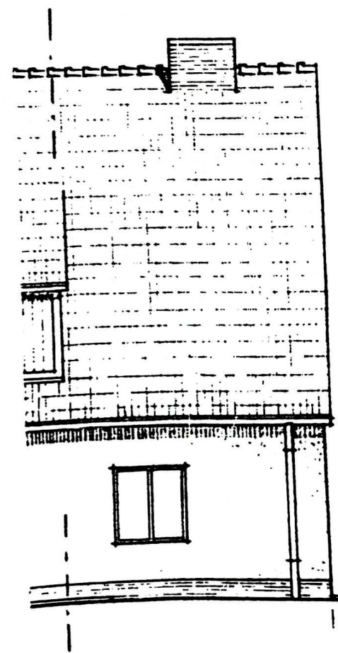
GARTENANSICHT
