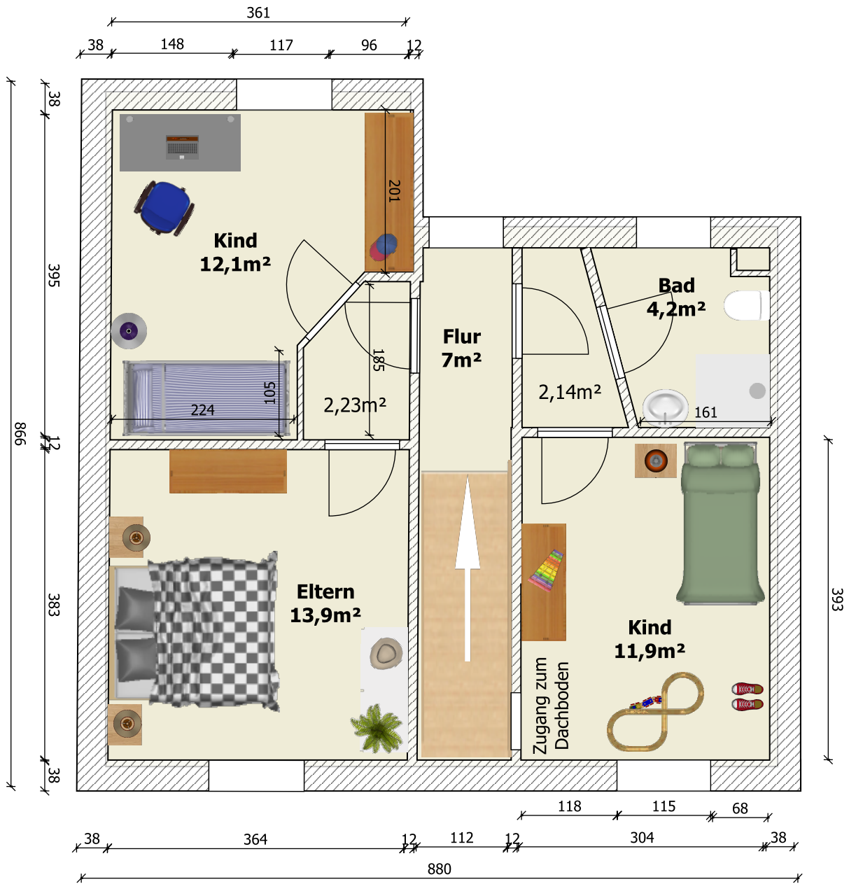
06237 Leuna, Schlosserstraße 17 Grundriss Obergeschoss Gestaltungsvorschlag
