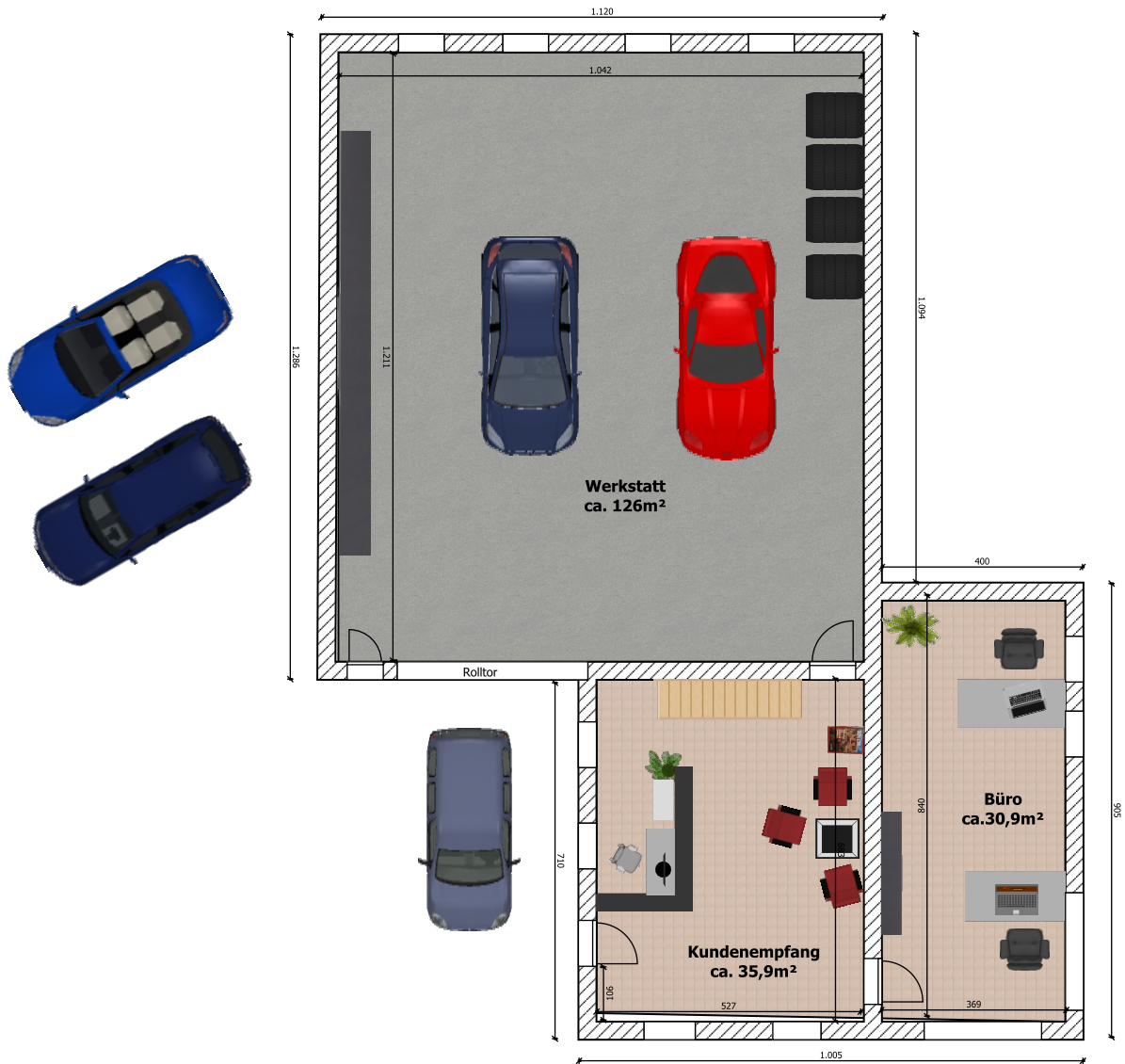
Rositz- Autowerkstatt, Grundriss Erdgeschoss www.wuestenrot-blk.de
