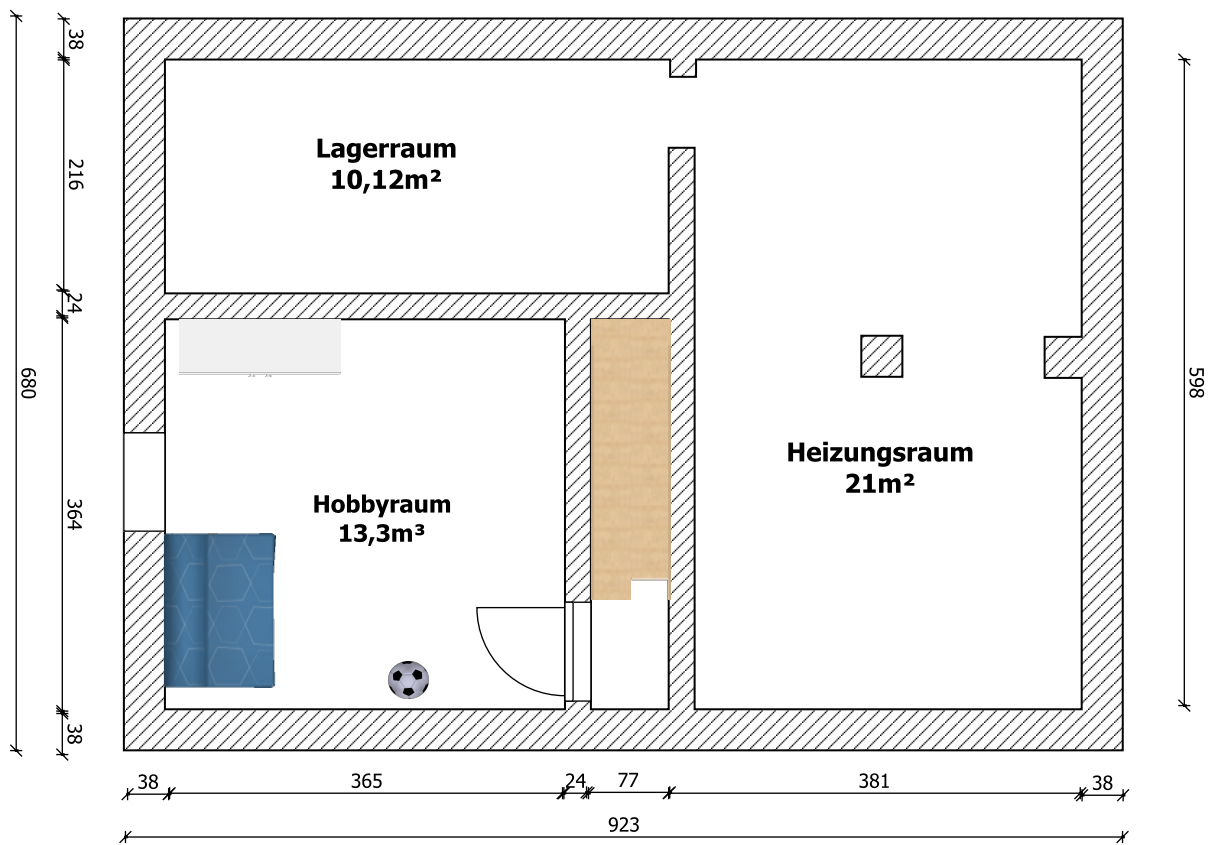
06237 Leuna, Schlosserstr.17 Grundriss Keller
