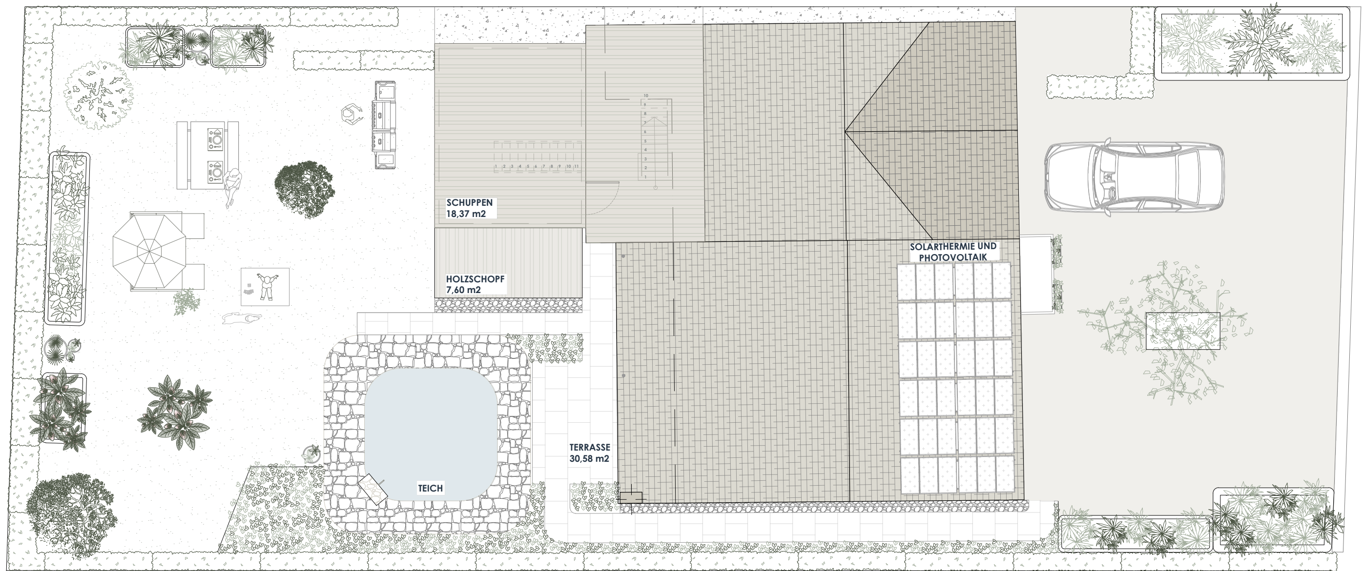
LAGEPLAN DES HAUSES AUF DEM GRUNDSTÜCK MIT BEMÄßUNG MAßSTAB/ 1.100
