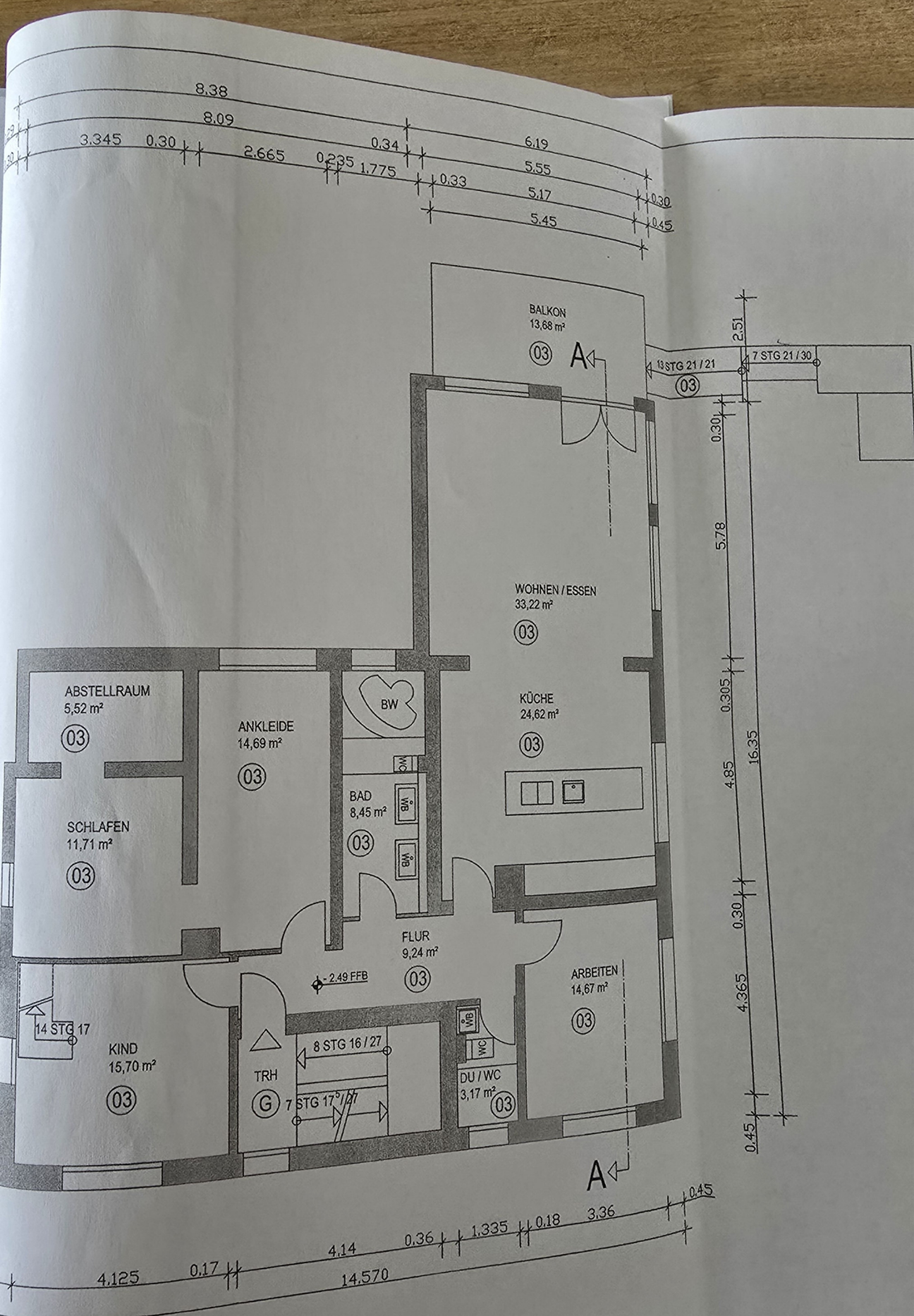
GRUNDRISS OBERGESCHOSS M:1:100
