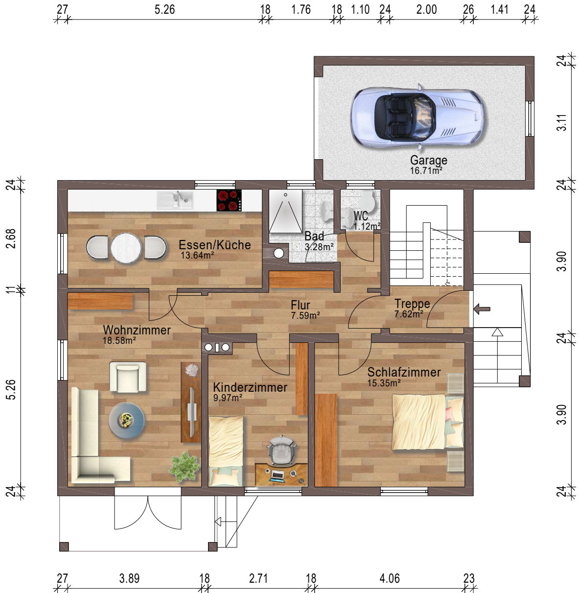
Erdgeschoss
