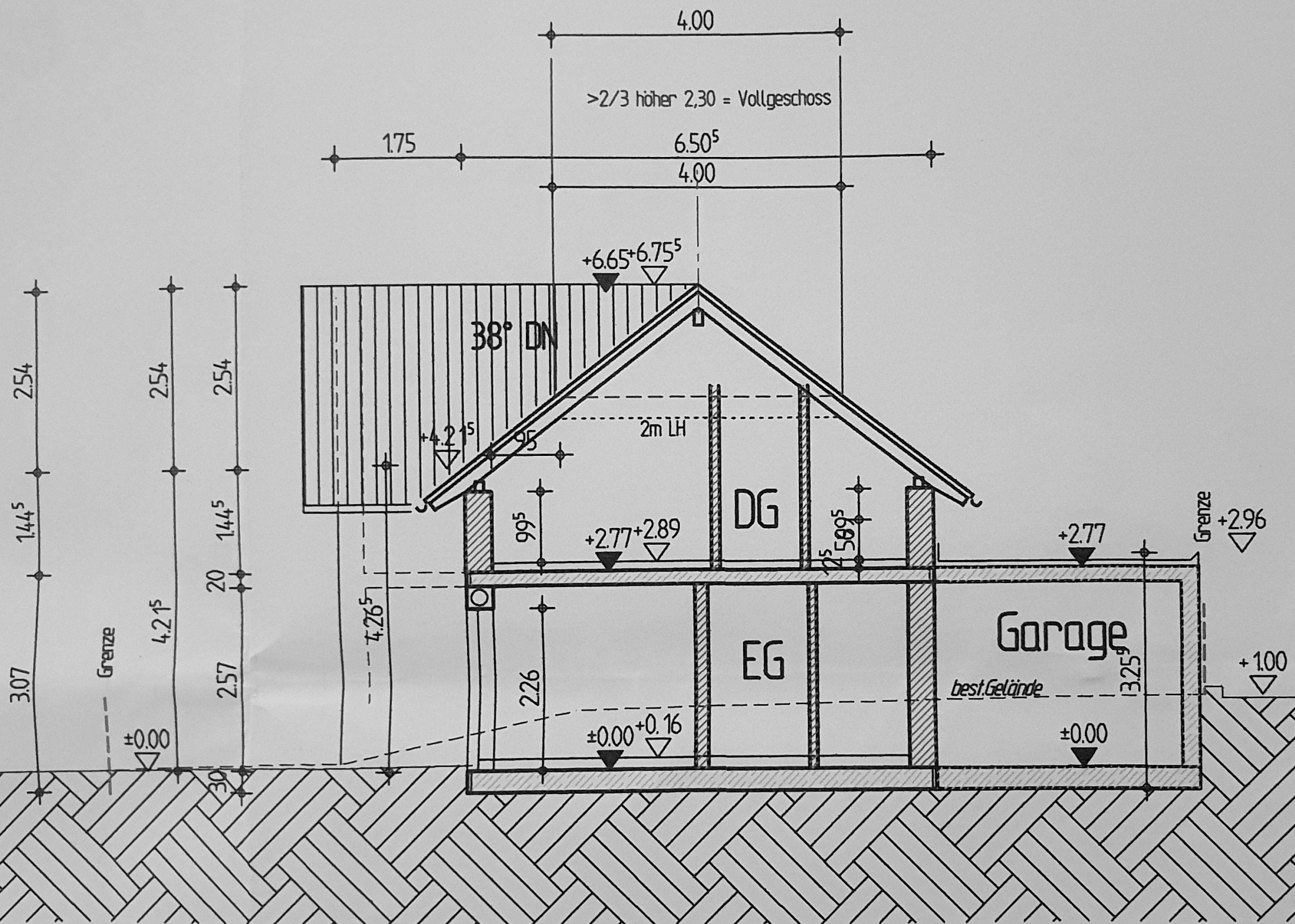
Schnitt A-A
