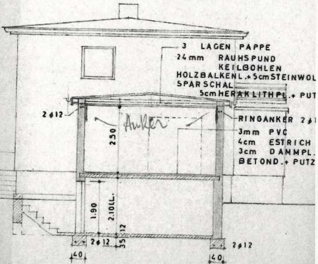
SCHNITT A-A 1:100
