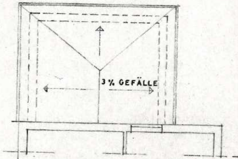
DACHAUFSICHT ANBAU 1:100
