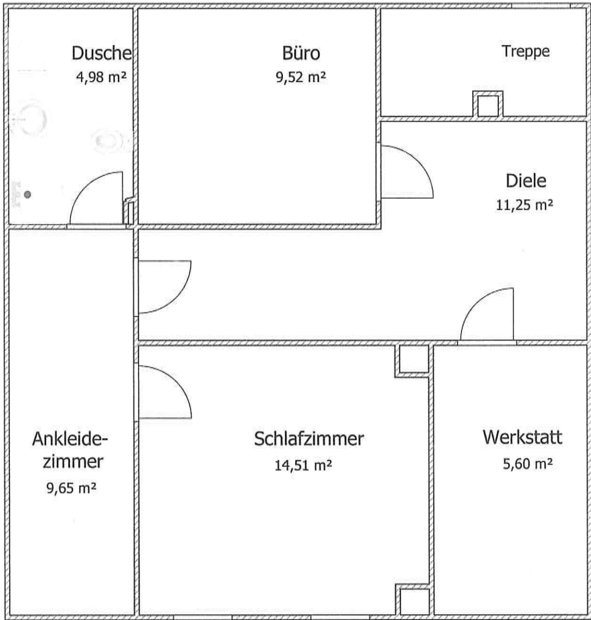
Grundriss Dachgeschoss
