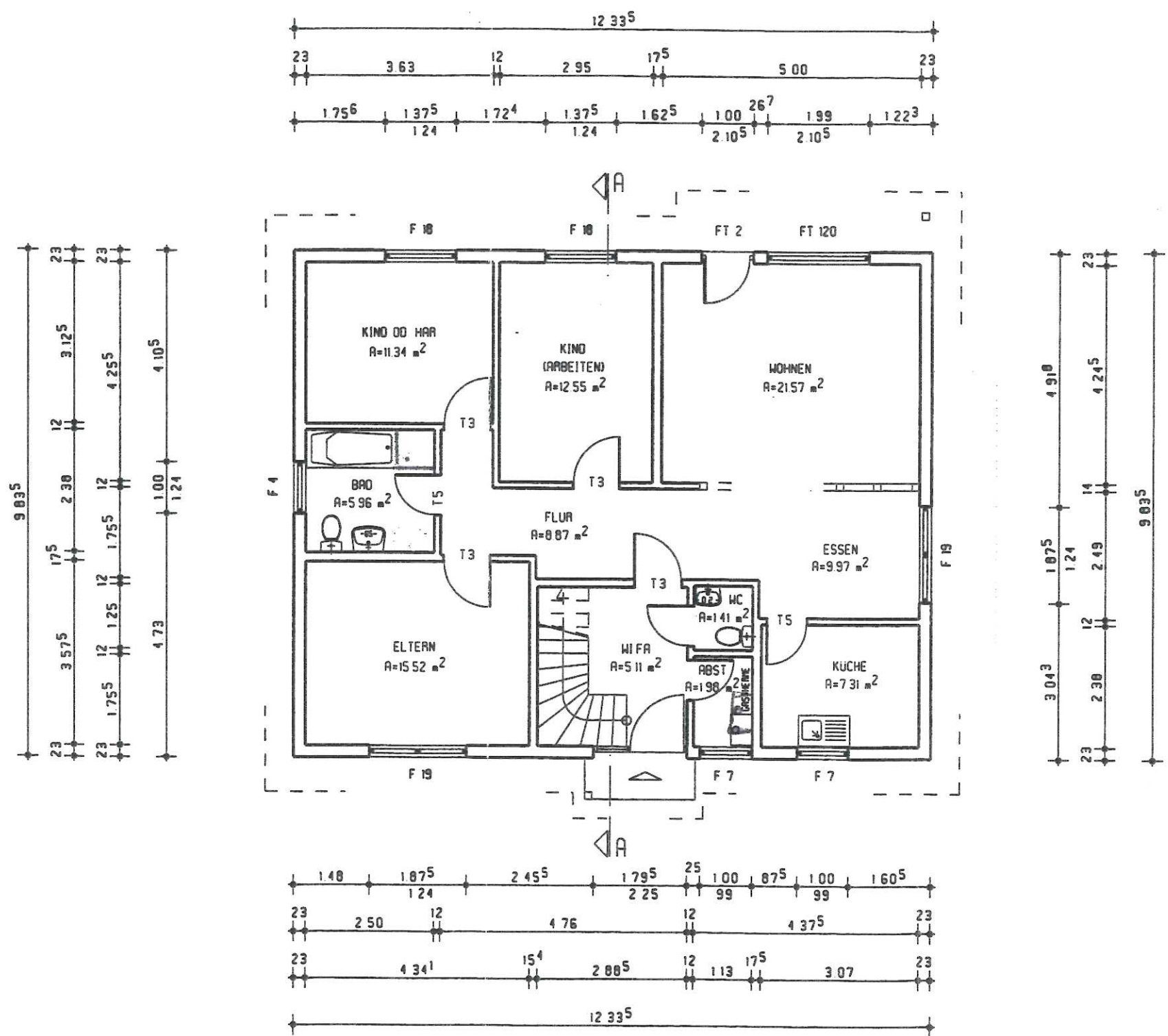
ERDGESCHOSS
