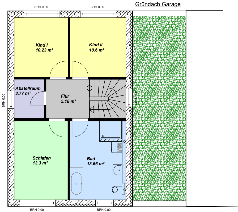
Endhaus 1.Obergeschoß
