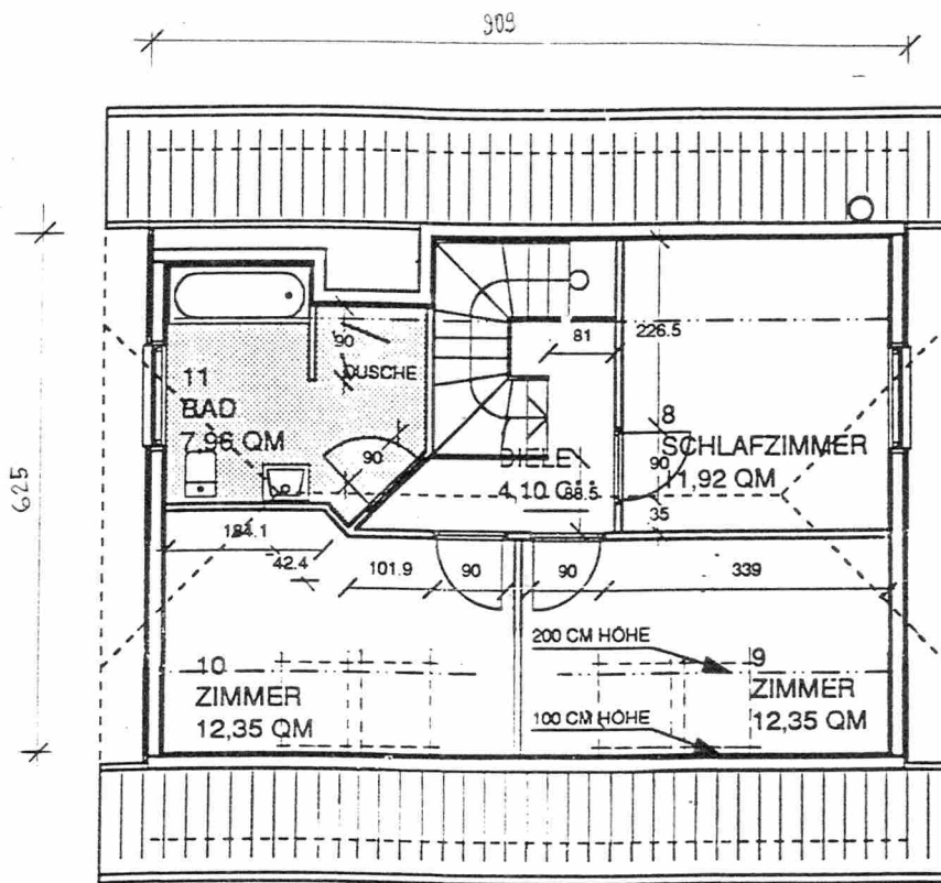
TYP 109 - DACHGESCHOß MAß 1 · 100
