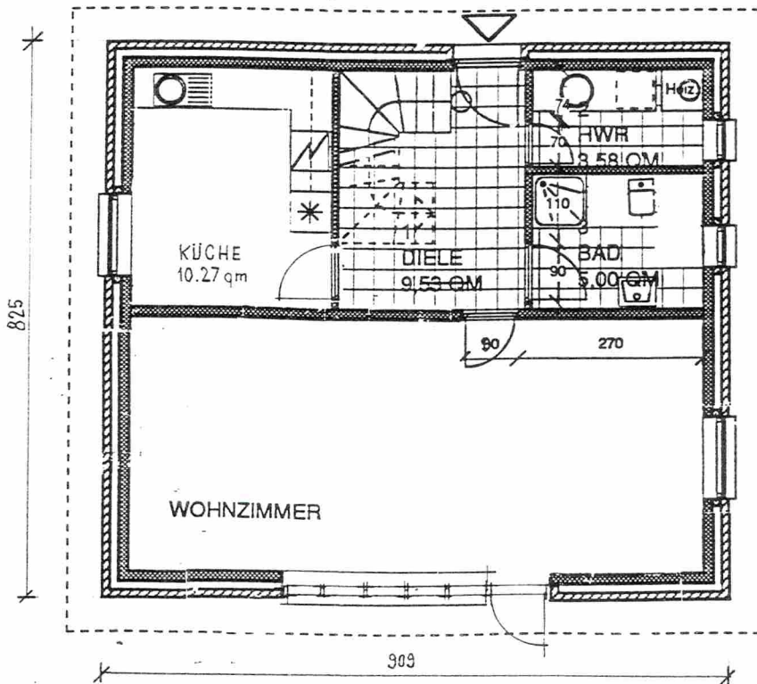
TYP 109 - ERDGESCHOß
