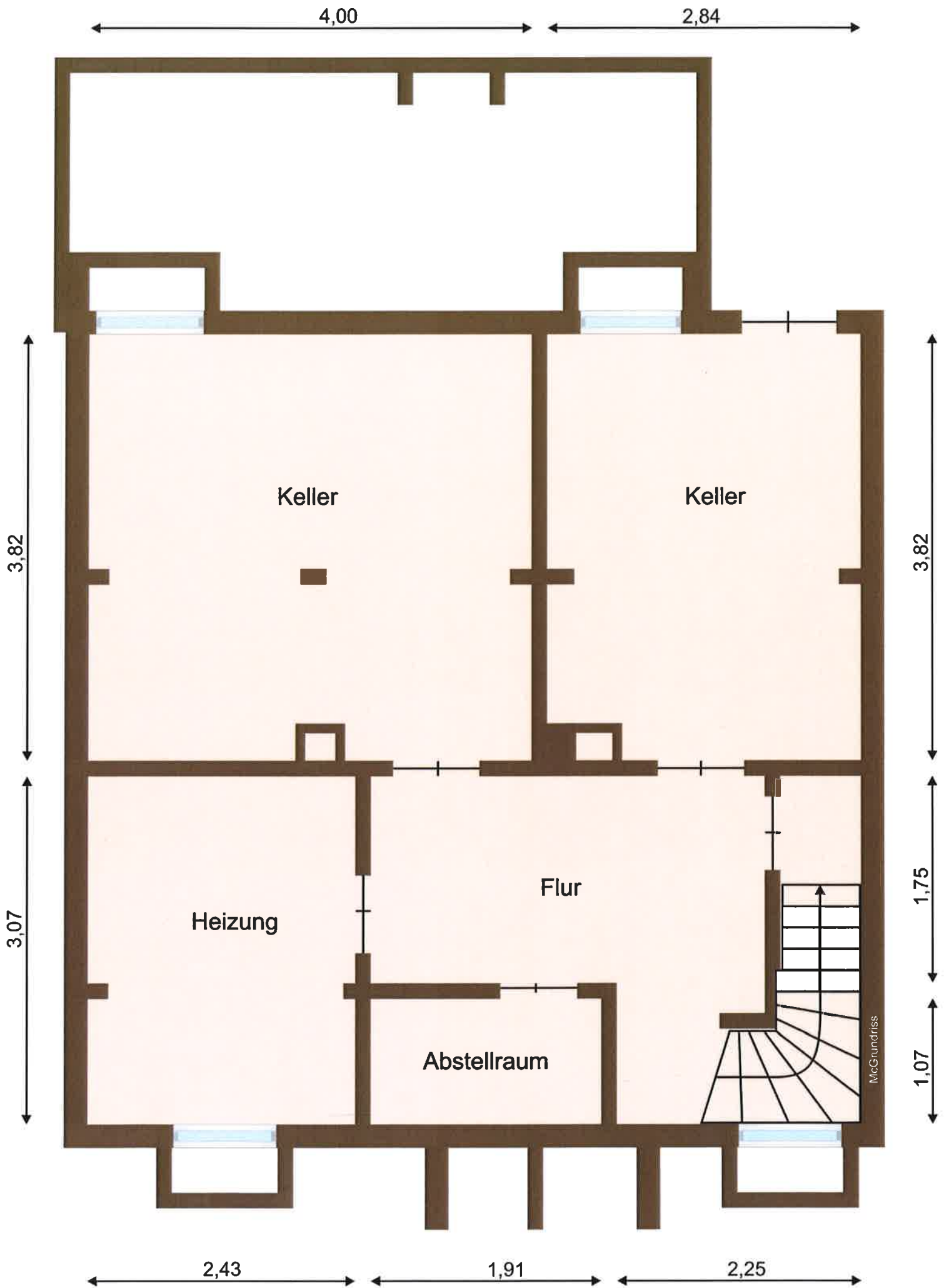
Kellergeschoss
