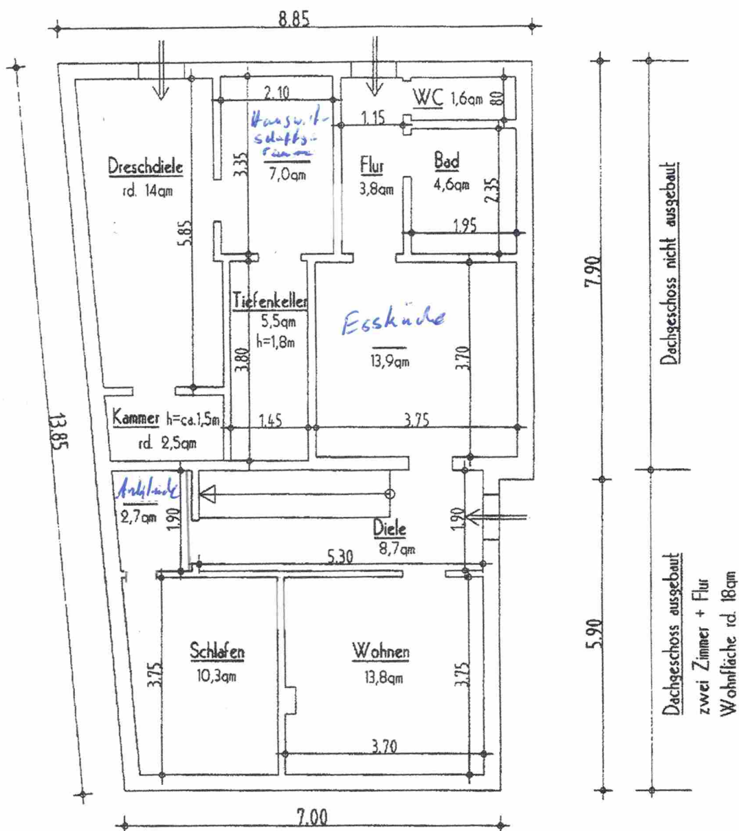
Grundriss EG
