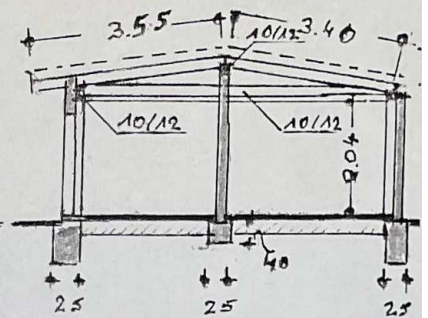
QUER SCHNITT
