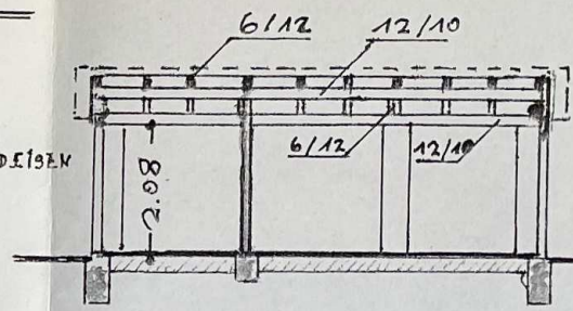
LÄNGEN SCHNITT
