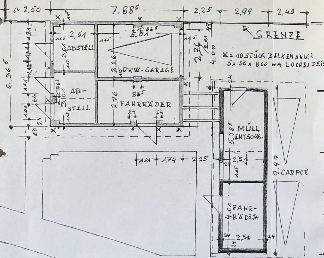
GRUNDRISS
