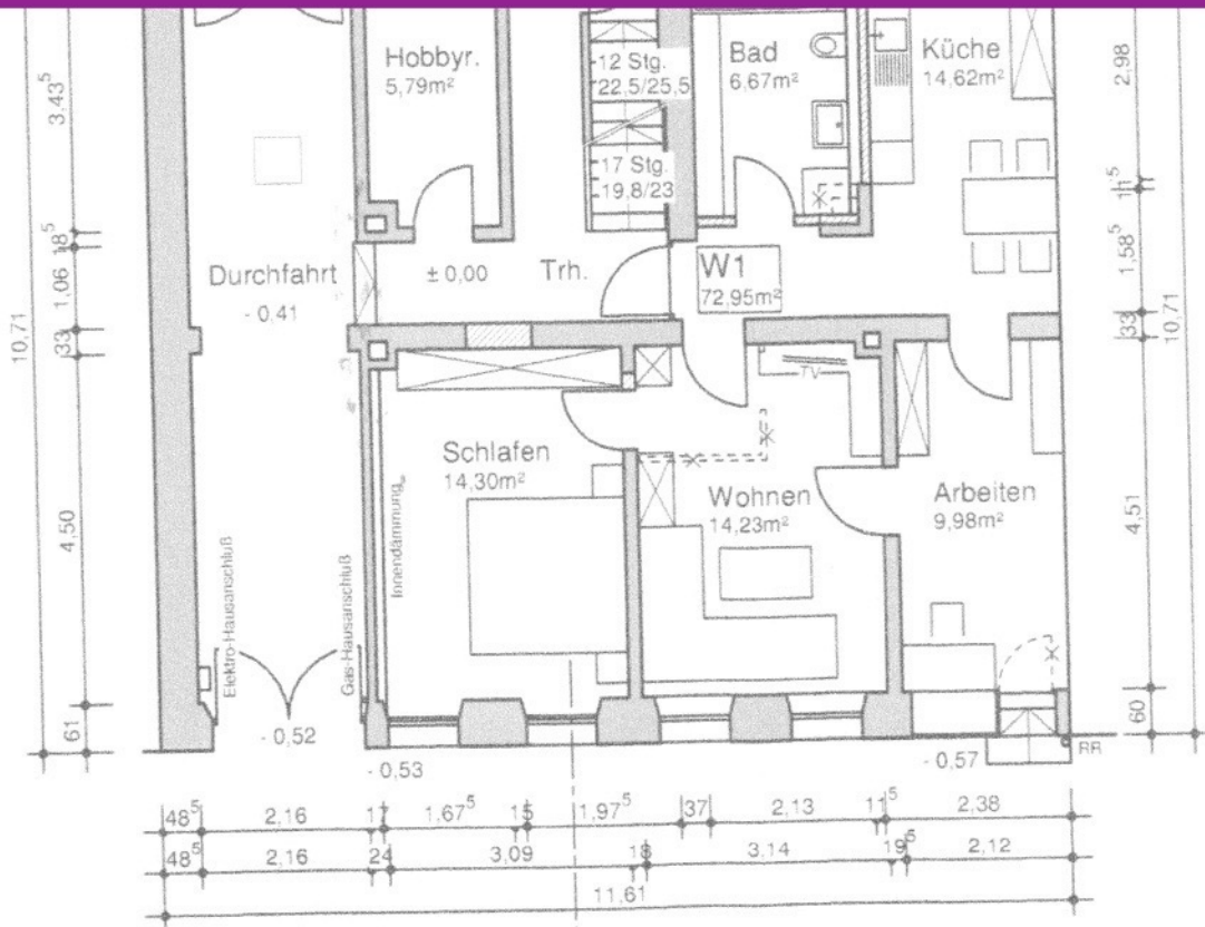
Erdgeschoss
