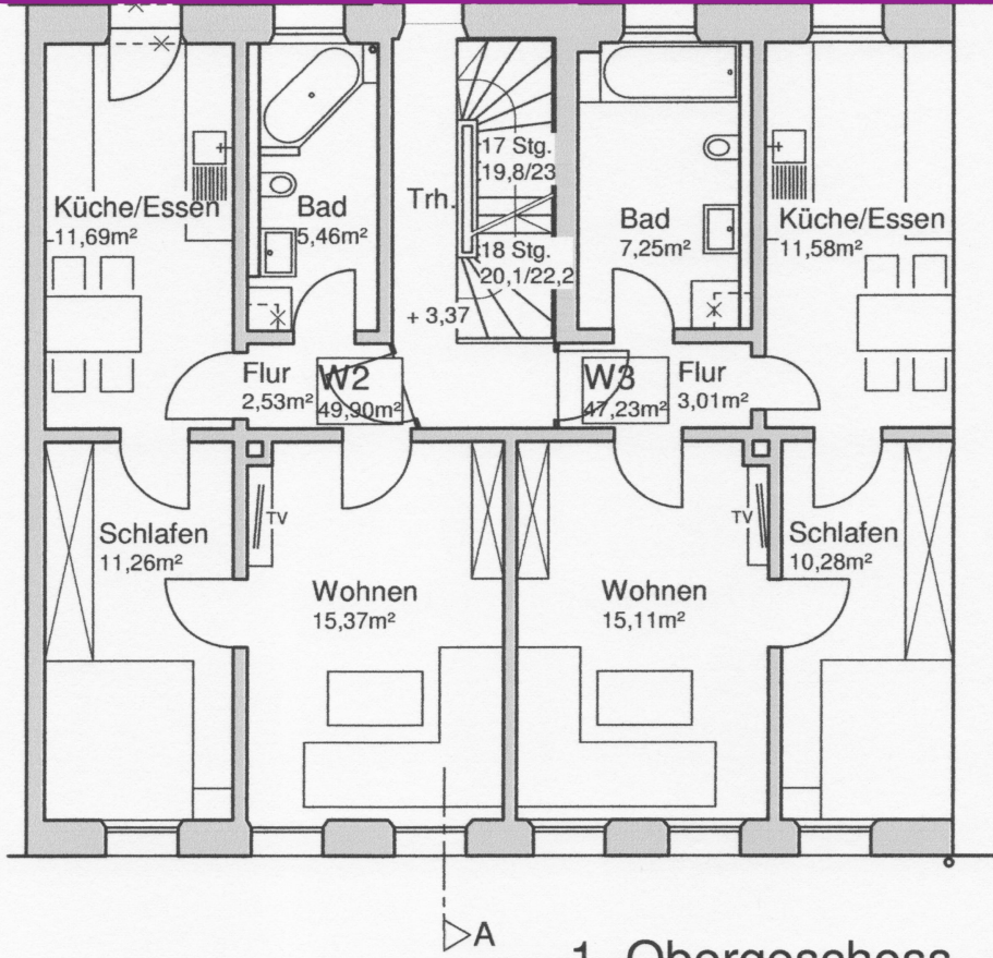
1. Obergeschoss
