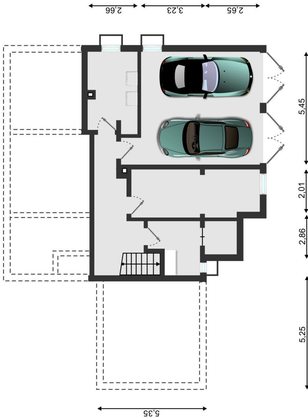
Kellergeschoss
