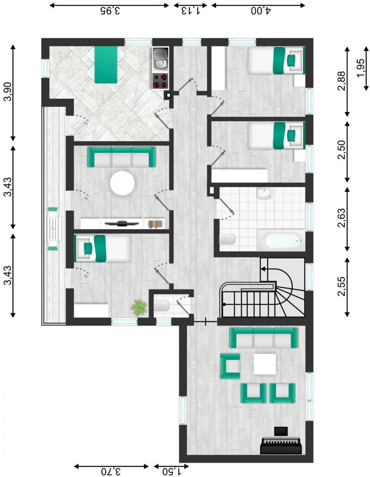
Obergeschoss
