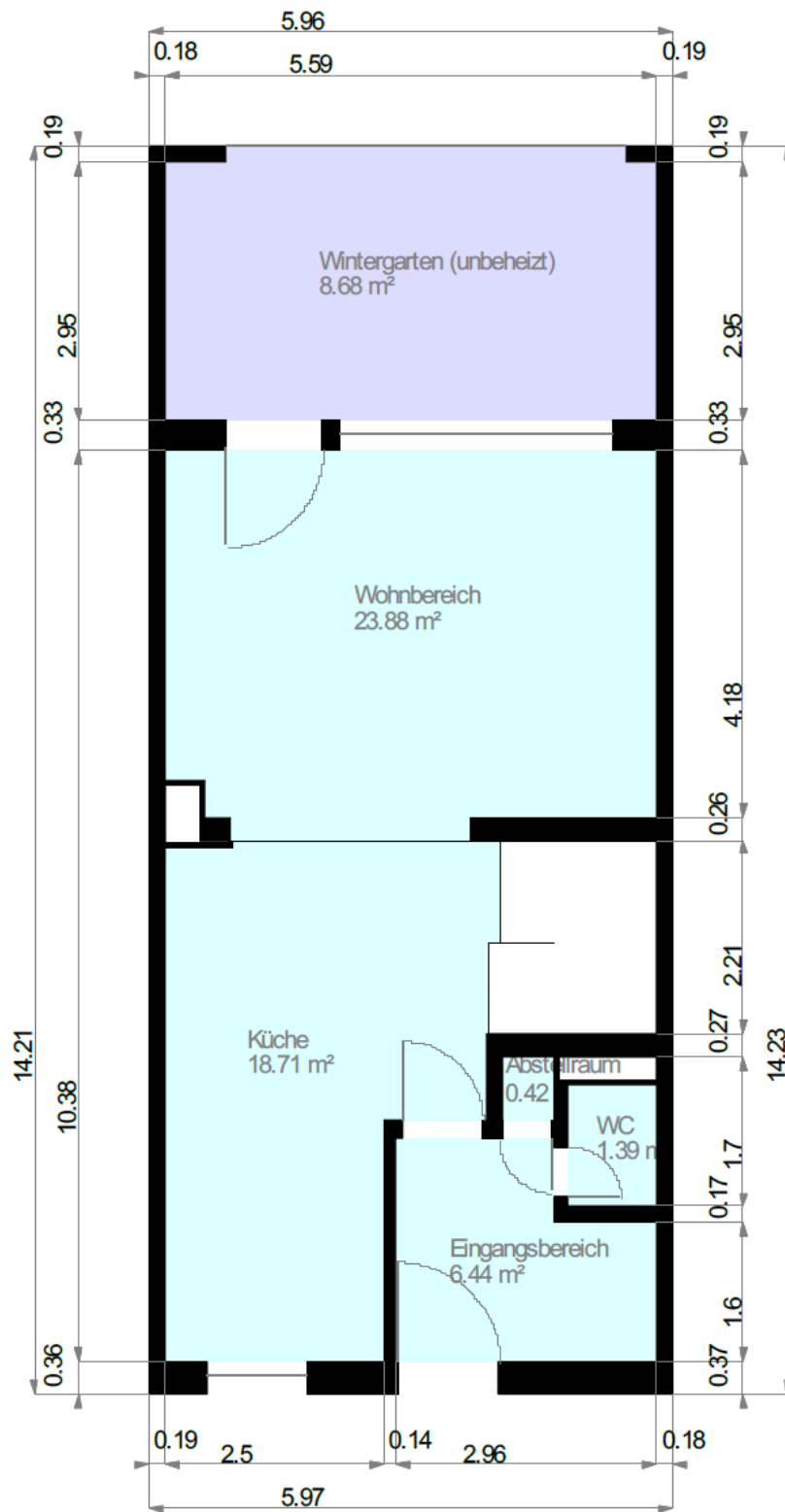
Erdgeschoss
