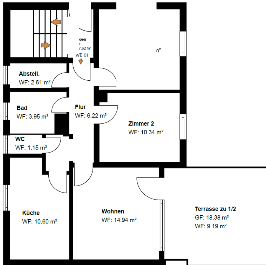
Erdgeschoss
