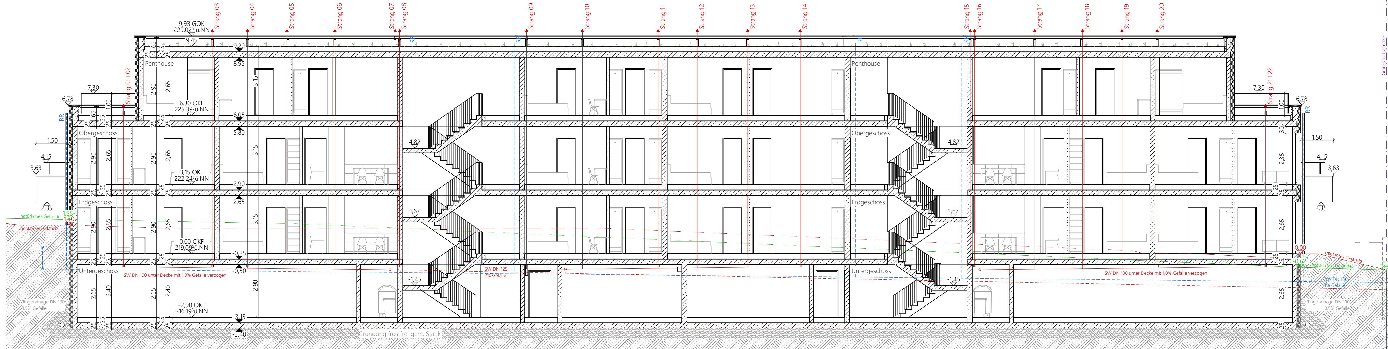
SCHNITT 01
