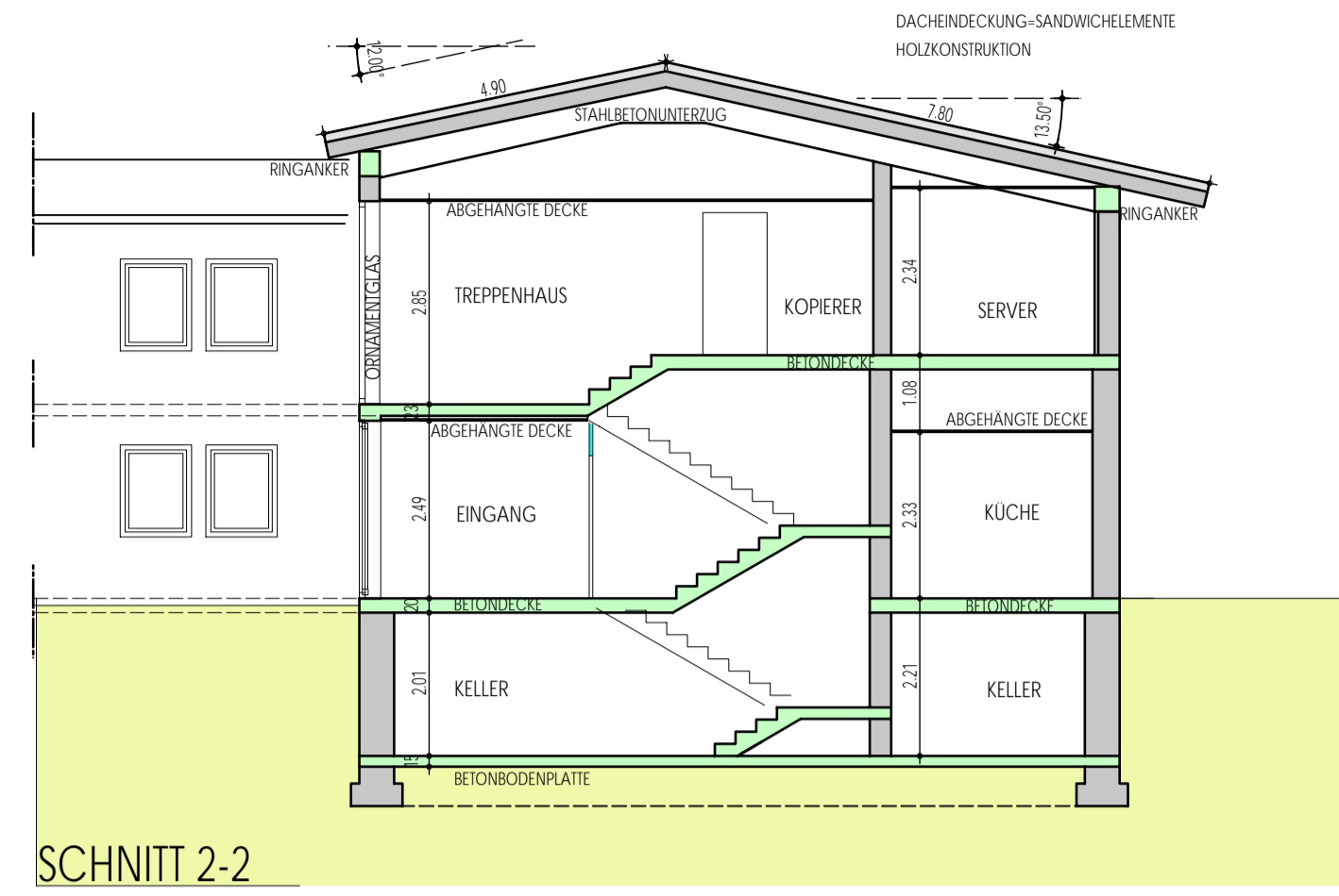
SNITT 2-2
