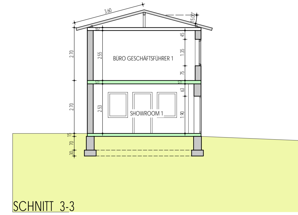
SNITT 3-3
