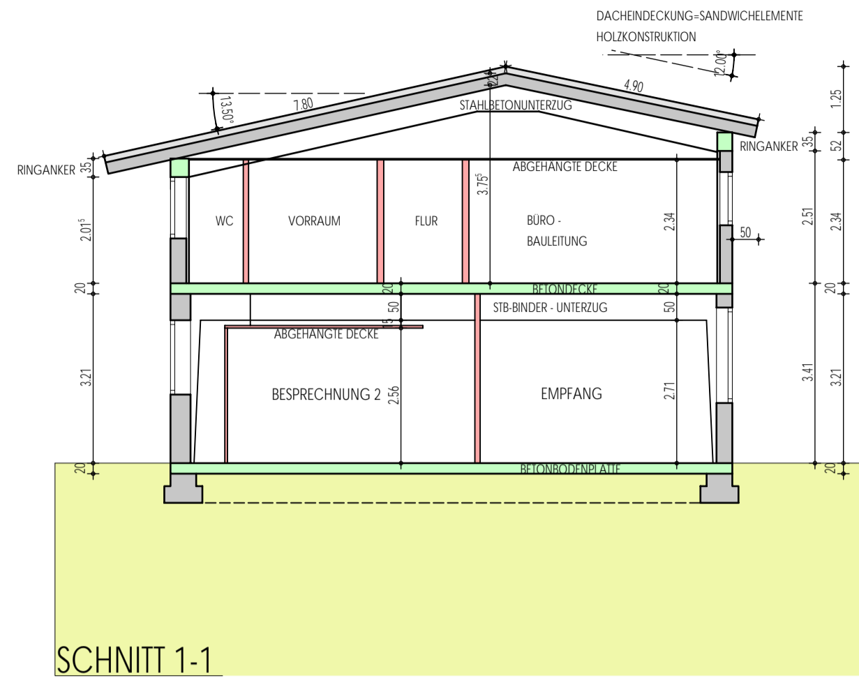
SNITT 1-1
