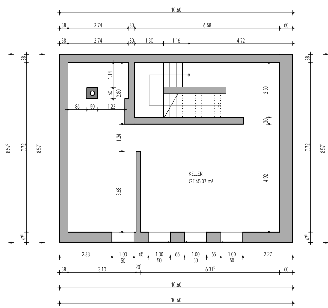
KELLERGESCHOSS
