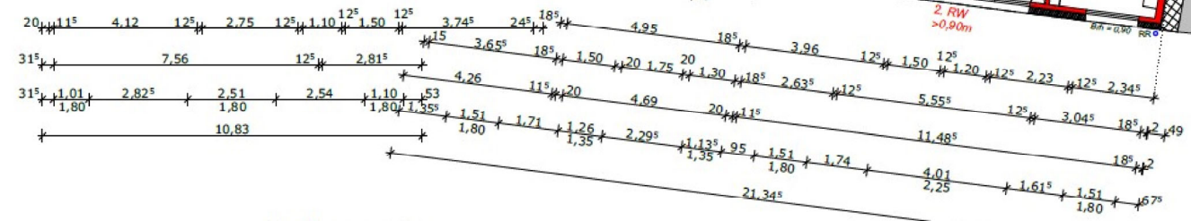
2. Obergeschoss
