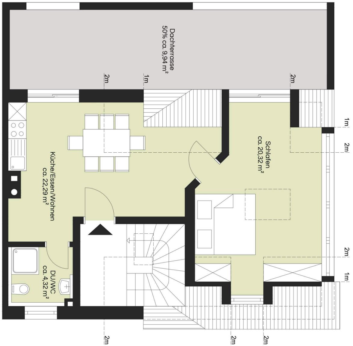
VARIANTE: AUSBAU DACHGESCHOSS MIT EINER EINLIEGERWOHNUNG
