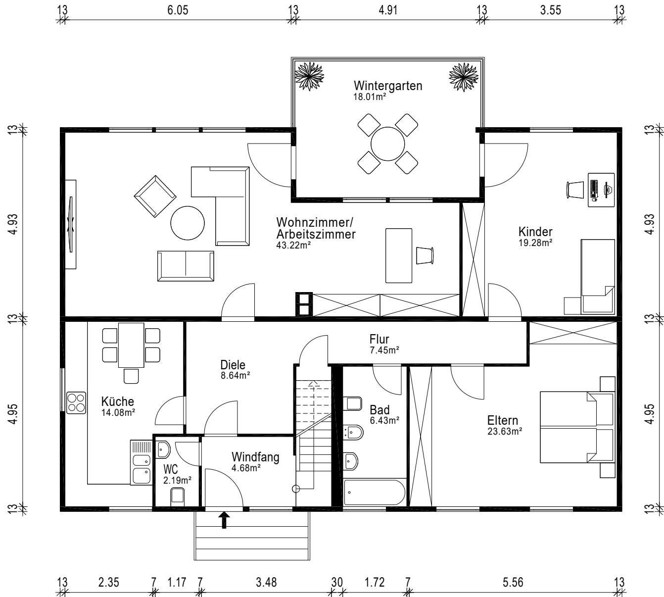
Erdgeschoss
